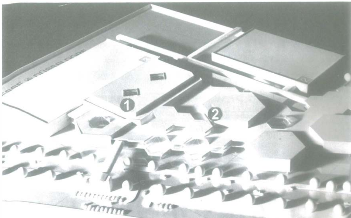
Die neue Stadthalle (1) liegt zwischen dem Messe-Congreß-Center (2) und zwei Messehallen. Links unten im Bild ist der überdachte Laufgang über die Rotterdamer Straße zu den Messeparkplätzen am Rhein zu sehen.
